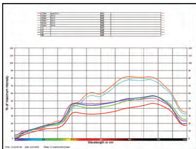
FIGURE 9. ½ fen VSC data.
